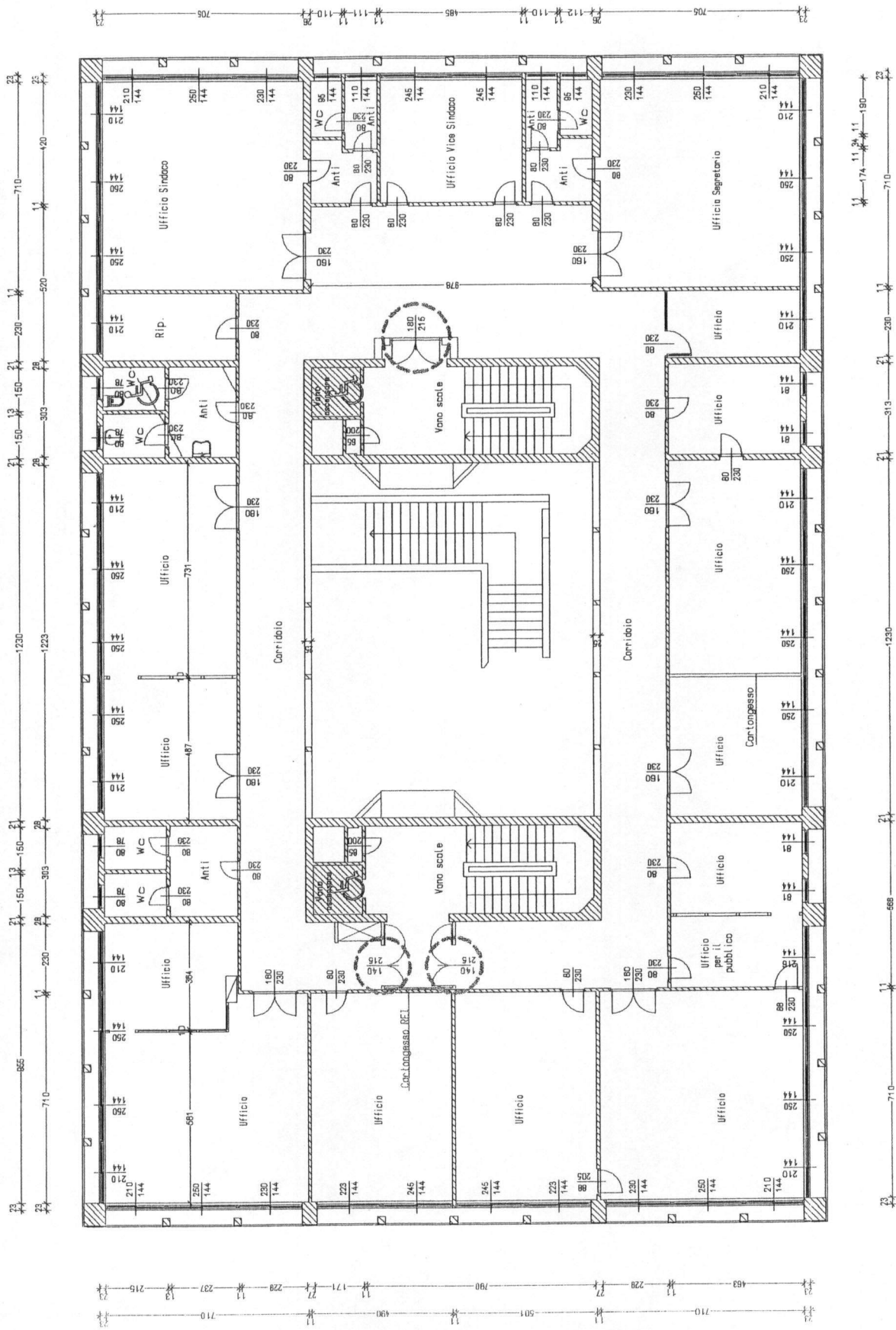
Pianta del piano Secondo h = 311 cm
