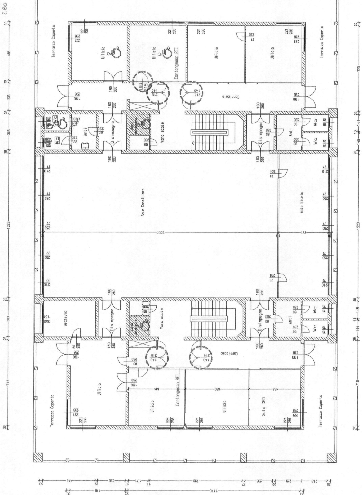
Pianta del piano Terzo h = 326 cm
